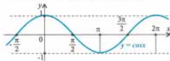
Grafiku i funksionit y = \cos x quhet kosinusoida .
